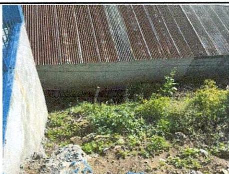
Foto 1: MEJORAMIENTO DE MURO DE CONCRETO CICLOPEO - Hay derrumbamientos del terreno de la escuela hacia la casa lo que provoca que la escuela no sea segura
